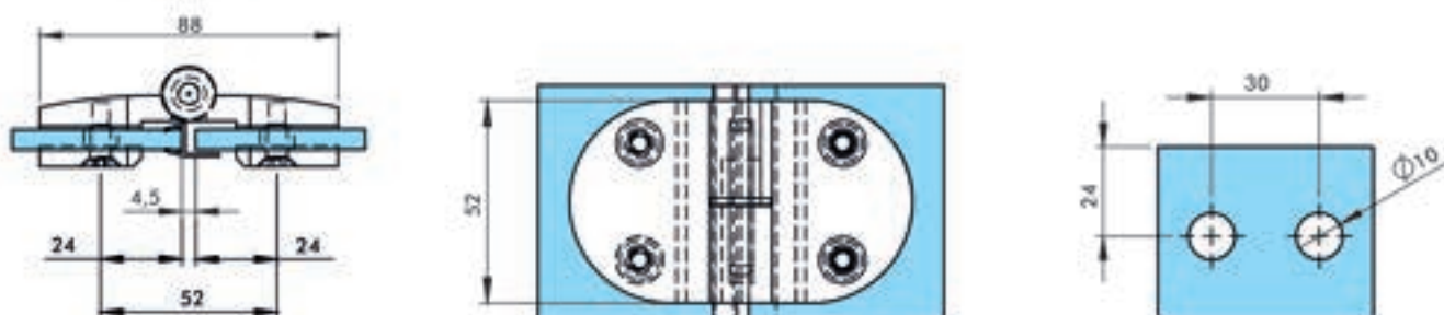
NY1-007 CAMDAN CAMA SAĞA - STEKLO K STEKLU YERNE, 180° dışarı açılır - открывается наружу NY1-008 CAMDAN CAMA SOLA - STEKLO K STEKLU SOLYA 180° dışarı açılır - открывается наружу 6-8 mm cam (Pirinç) - стекло (latuya)
