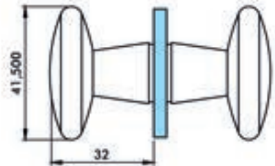
NY2-002 KAPİ KOLU YUVARLAK - ДВЕРНАЯ РУЧКА КРУГЛАЯ Değiş çapı - Диаметр отверстия 10 mm, 6-8-10 mm çap (Fıncık) - стекло (пагуна)
