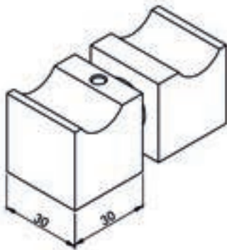
NY2-014 KAPİ KOLU - ДВЕРНАЯ РУЧКА Delik çapı - Диаметр отверстия 10 mm, 6-8-10 mm cam (Alüminyum) - стекло (Алюминий)
