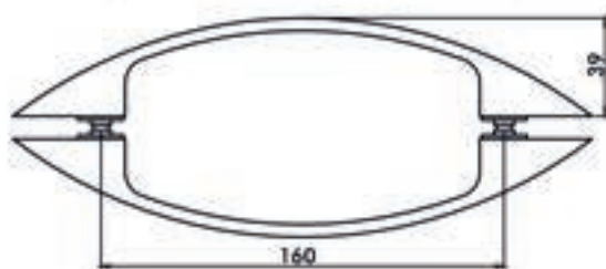
HY2-302 KAPLI KOLU - ДВЕРНАЯ РУЧКА LO:160 mm Delik çarı - Диаметр отверстия 10 mm, 6-8-10 mm çam (Çirko) - стекло (çine)
