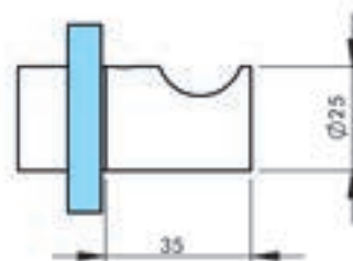
NY5-004 TEKİ CAM BAĞLANTI - СОЕДИНЕНИЕ ОДНОГО СТЕКЛА Değiş çap - Диаметр отверстия 10 mm 6-8-10 mm cam (Piring) - стекло (палюва)
