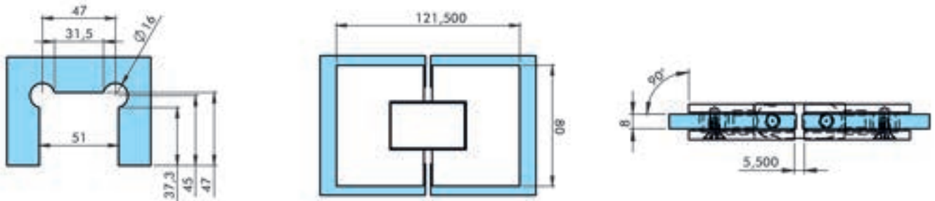
HY1-084 SANDAN SAMA YAY - ПРУЖИНА СТЕКЛО-СТЕКЛО Tek taraflı 90° açılır. - Одностороннее открытие на 90°. 6-8-10 mm cam (Çinko) - стекло (cam)
