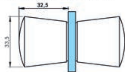
NY2-004 KAPİ KOLU FİTA - ДВЕРНАЯ РУЧКА ФИТА Değiş çapı - Диаметр отверстия 10 mm, 6-8-10 mm çap (Çap) - стекло (Цанк)
