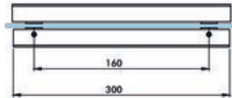
NY2-019 KAPİ KOLU - ДВЕРНАЯ РУЧКА L0:160 L:300 mm Delik çapı - Диаметр отверстия 9 mm, 6-8-10 mm cam (Alüminyum) - стекло (Алюминий) (L0.X L.X mm) Her boyutta üretilmiştir - Изготавливается во всех размерах
