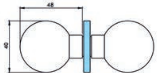
NY2-003 KAPİ KOLU KRİSTAL - ДВЕРНАЯ РУЧКА КРИСТАЛЛ Değiş çapı - Диаметр отверстия 10 mm, 6-8-10 mm çap (Çap) - стекло (Стекло)
