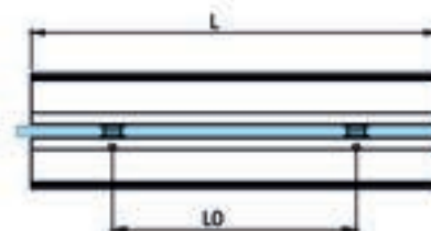
NY2-022 KAPİ KOLU - ДВЕРНАЯ РУЧКА L0:160 L:300 mm NY2-023 KAPİ KOLU - ДВЕРНАЯ РУЧКА L0:30 L:50 mm Delik çapı - Диаметр отверстия 9 mm, 6-8-10 mm cam (Fırınç) - стекло (латунь) (L0.X L.X mm) Her boyutta üretilmiştir - Изготавливается во всех размерах
