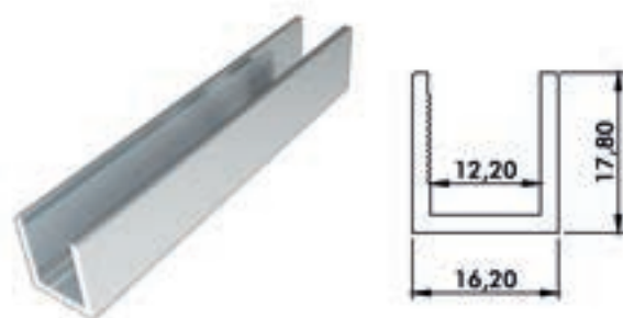
HY9-041 PROFİL - ПРОФИЛЬ U 18*16 Alüminyum - Alüminyum
