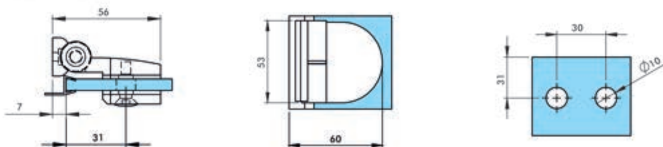
NY1-009 DUVARDAN CAMA SAĞA - OT STENY K STEKLU YERNE, 90° dışarı açılır - открывается наружу NY1-010 DUVARDAN CAMA SOLA - OT STENY K STEKLU SOLYA 90° dışarı açılır - открывается наружу 6-8 mm cam (Pirinç) - стекло (latuya)
