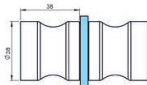
NY2-011 KAPİ KOLU DÜZ - ДВЕРНАЯ РУЧКА ПРЯМАЯ Deñik çapı - Диаметр отверстия 10 mm, 6-8-10 mm çam (Pirinç) - стекло (пазлы)
