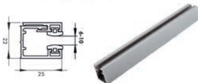
HY9-017 PROFİL 22*15 CONTACT - ПРОФИЛЬ 22*15 ПРОКЛАДочный , Krom - Krom 6-8-10 mm cam (Alüminyum) - cam (Alüminyum)
