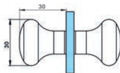
NY2-013 KAPİ KOLU RÜSTİK - ДВЕРНАЯ РУЧКА РУСТИК Deñik çapı - Диаметр отверстия 10 mm, 6-8-10 mm çam (Pirinç) - стекло (пазлы)
