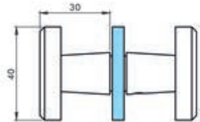
NY2-001 KAPİ KOLU KARE - ДВЕРНАЯ РУЧКА КВАДРАТНАЯ Değiş çapı - Диаметр отверстия 10 mm, 6-8-10 mm çap (Fıncık) - стекло (пагуна)
