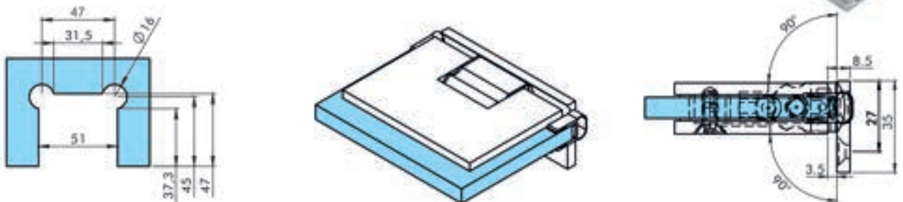
HY1-085 WALL TO GLASS SPRING Her iki taraflı 90° açılabilir. - Обе стороны открываются на 90°. 6-8-10 mm cam (Çinko) - стекло (cam)
