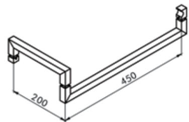
HY2-520 DOOR HANDLE LO:200 LO:450 mm Hole diameter 10 mm, 6-8-10 mm glass (Brass)
